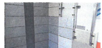
Platten aus Materialien wie Granit, Marmor, Keramik und Dekton, alle befestigt mit dem Verankerungssystem Keep-nut von Specialinsert Foto: Firma
